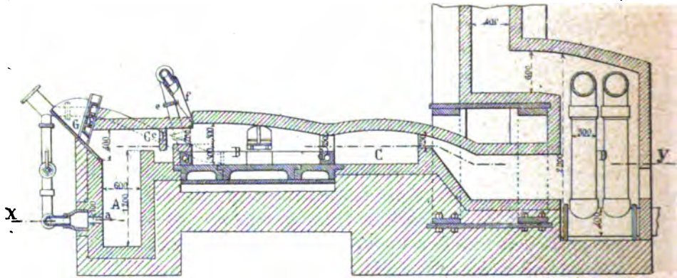
Coupe XY
